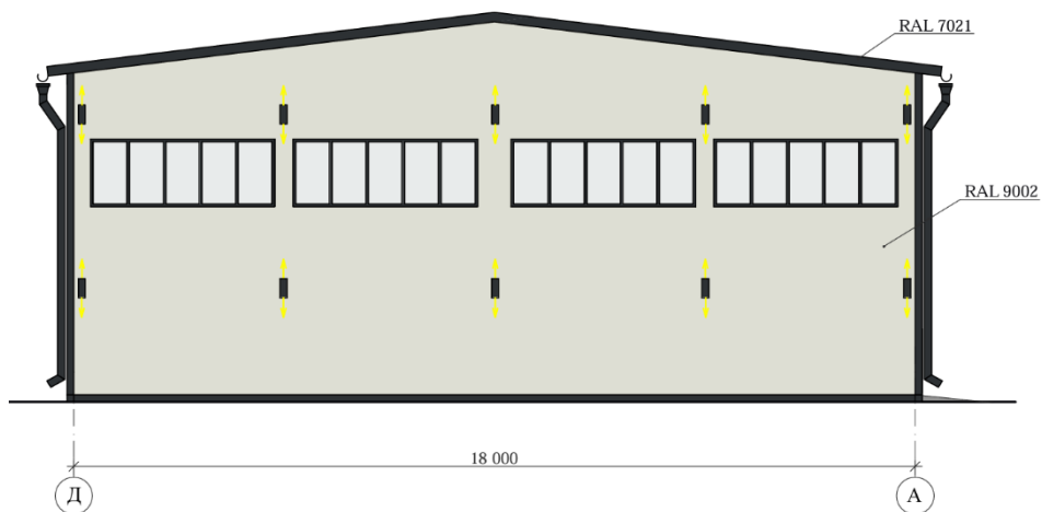
Фасад в осях Д-А
