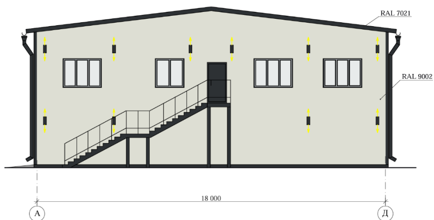
Фасад в осях Д-А
