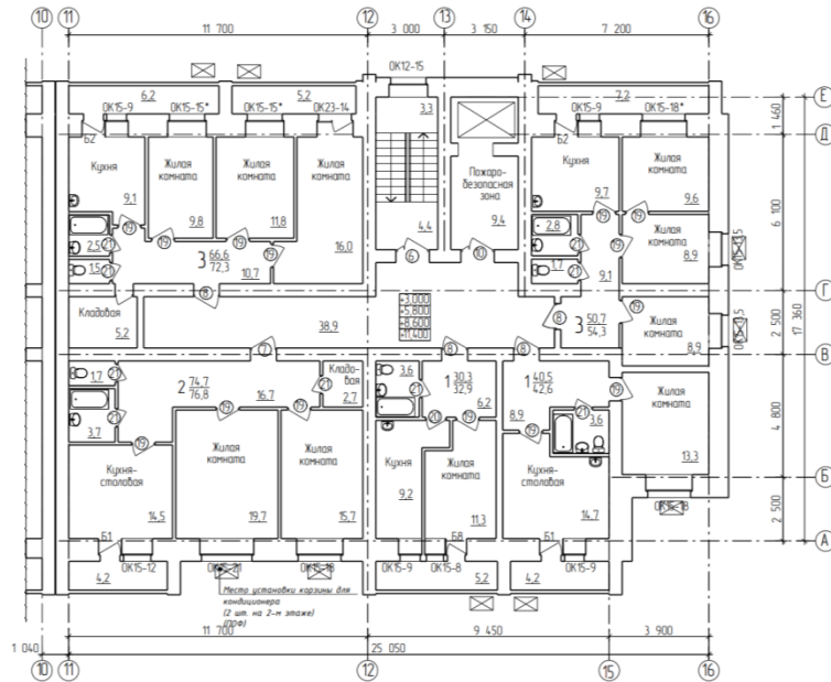
План 6-го - 10-го этажей между осями 1-10
