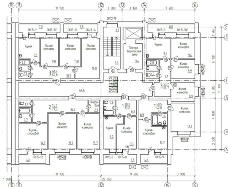
План 6-го - 10-го этажей между осями 11-16
