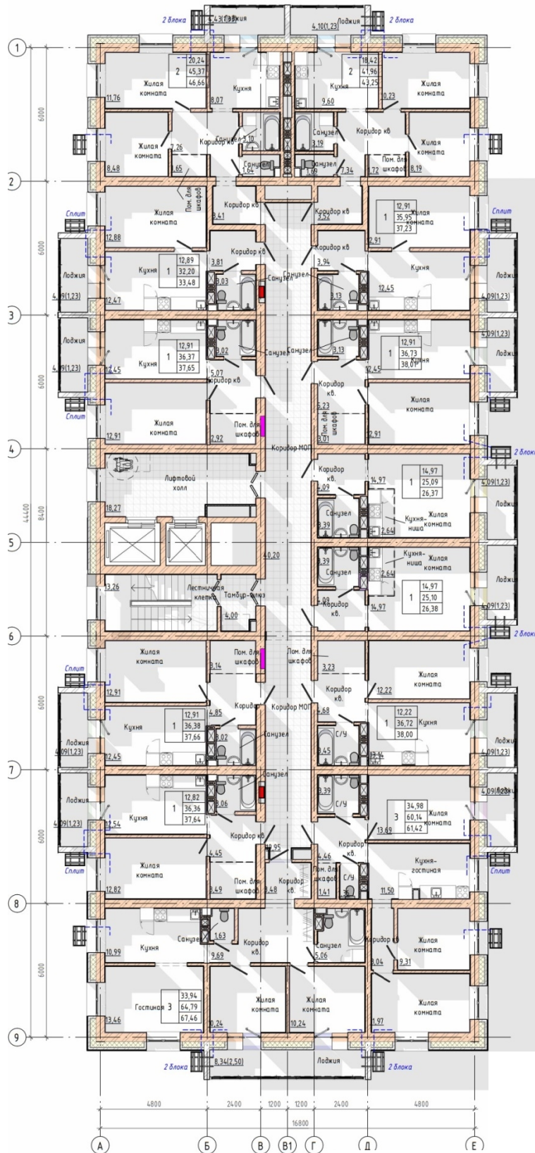
План типового этажа на отм. +4,500...+31,500
