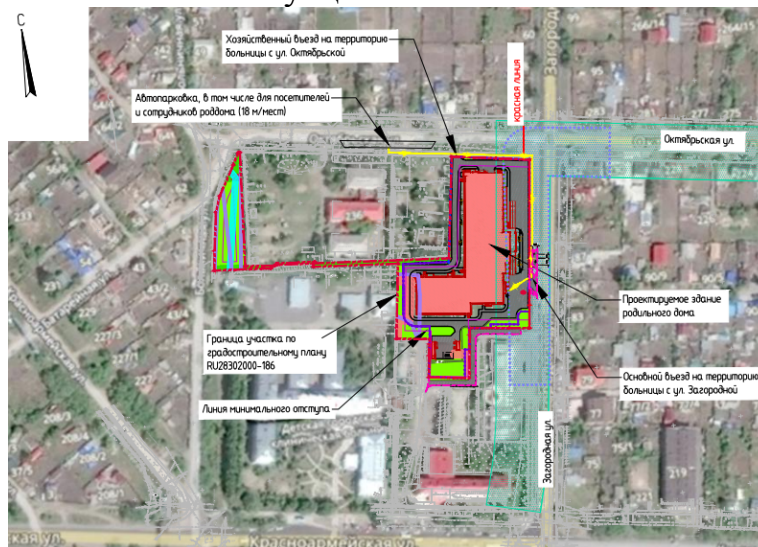
ситуационный план
