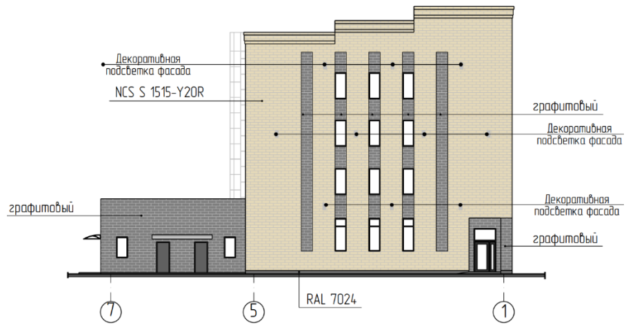
Фасад 7-1
