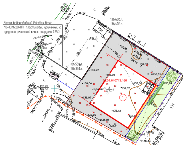
План застройки
