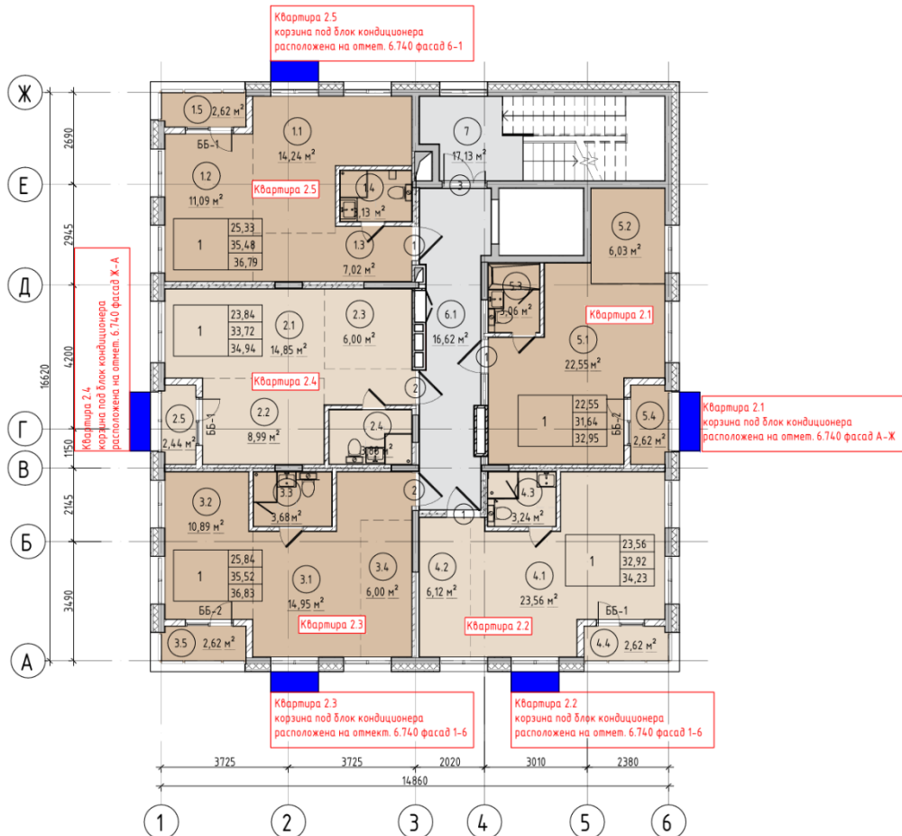
План расположения корзин под внешние блоки кондиционеров для квартир 2 этажа
