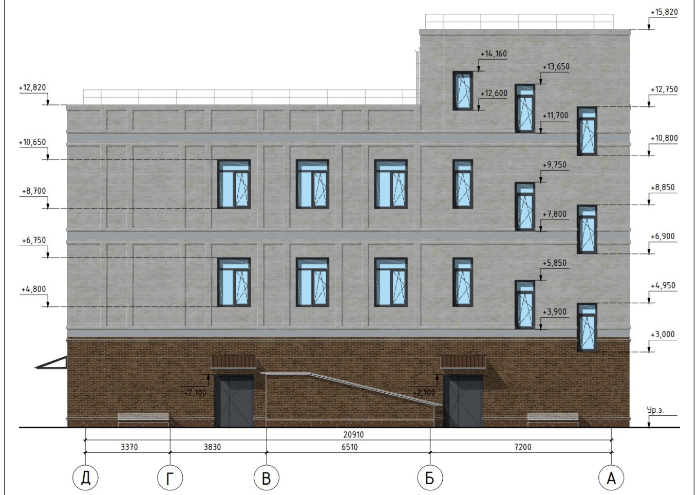
Фасад Д-А
