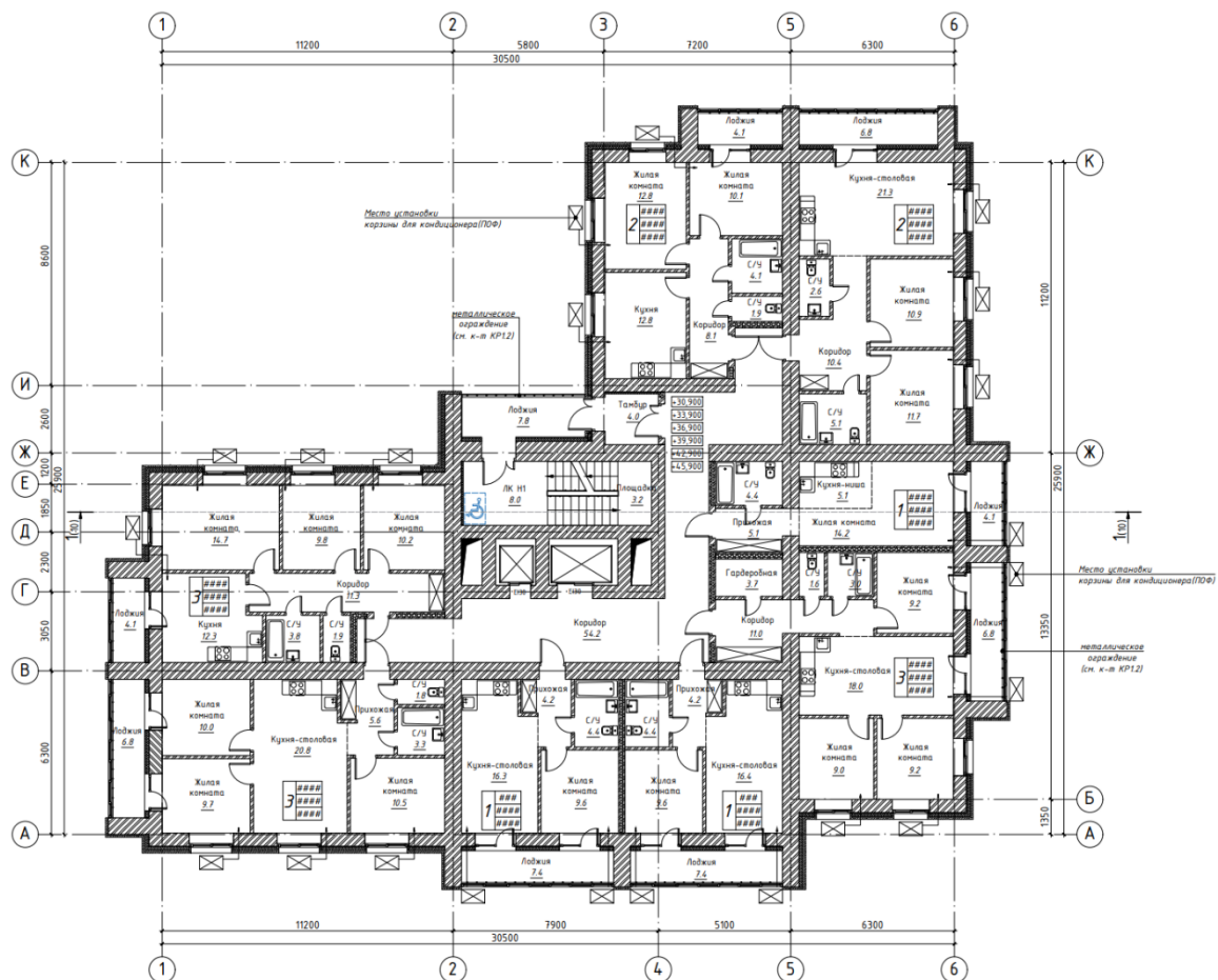
План 11-го - 16-го этажей
