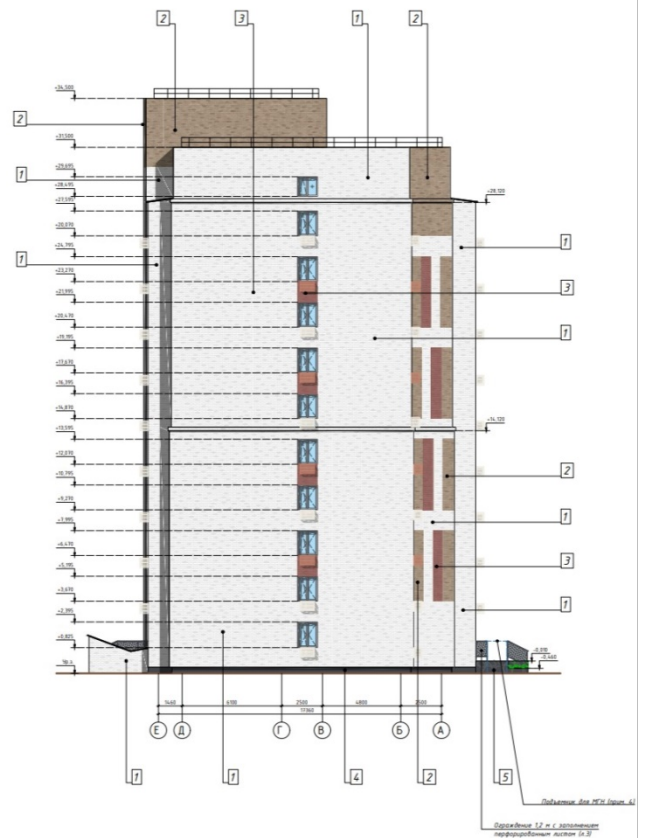
Фасад А-Е
