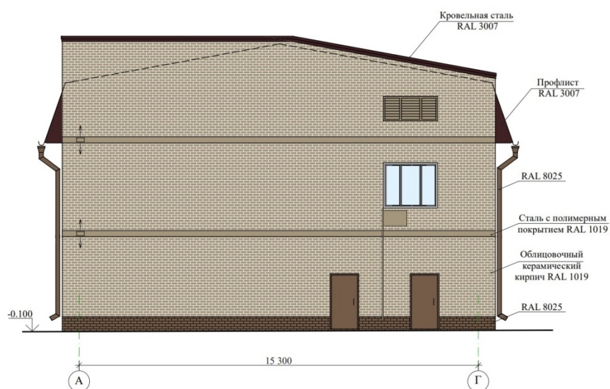
Фасад А - Г
